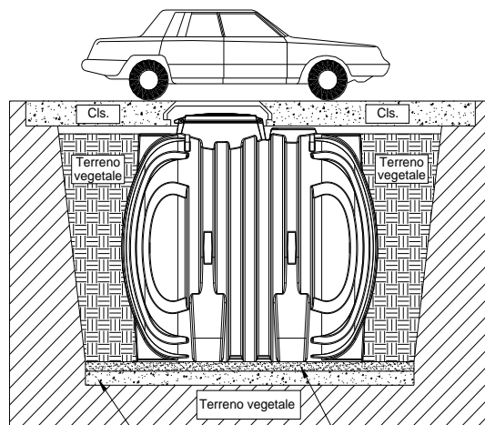
FIG. 3.1 Soletta in cls Letto di sabbia
