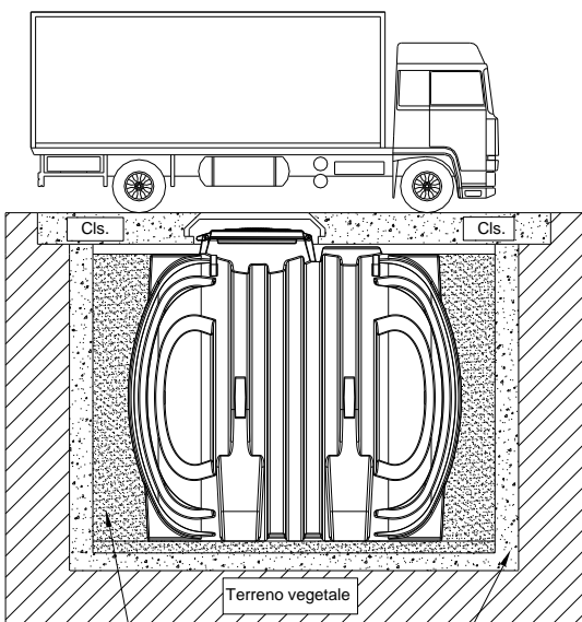
FIG. 3.2 Sabbia Cassaforma in cls. armato
